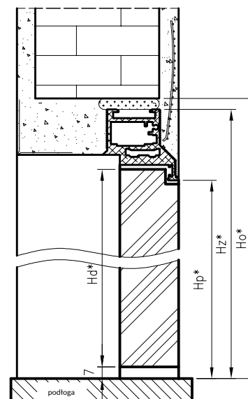
Przekrój pionowy drzwi Sara Eco 2 przylgowe - otwierane do wewnątrz
